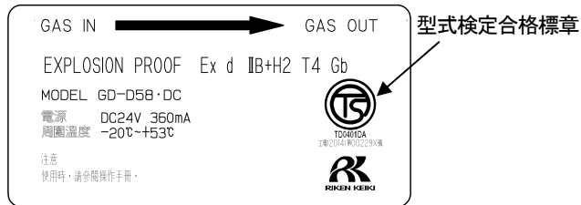
Taiwan Ex (TS) 仕様の銘板例 (AC/DC 電源仕様)
